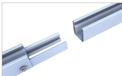
Expansionsskarv C47 S för profilklamrar
