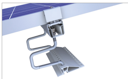
Dubbeltakkrok för höga snöbelastningar
